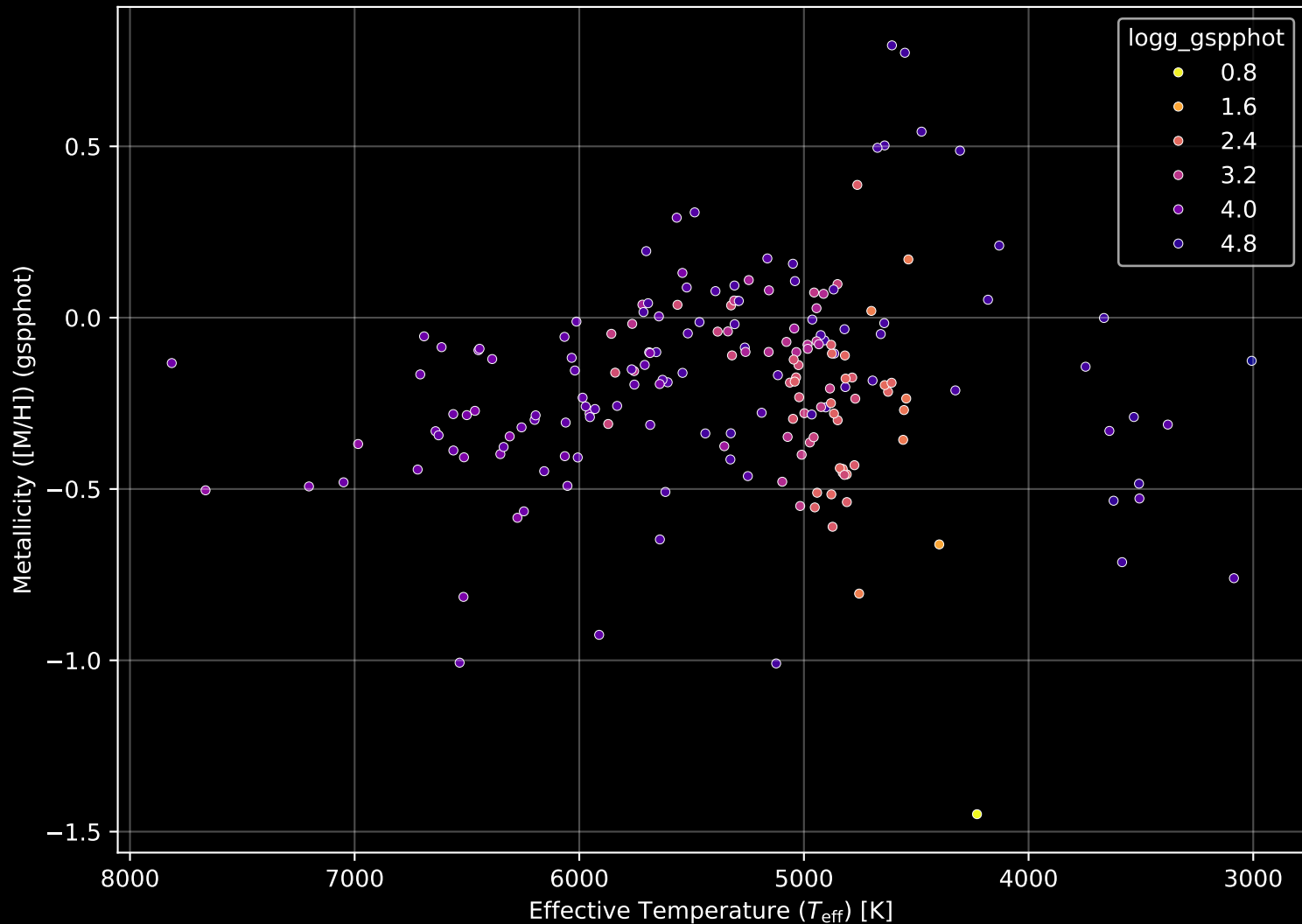
APOGEE DR17 Field: [CVZTILE_103+38_btx] Stellar Population Parameters (n= 193)
